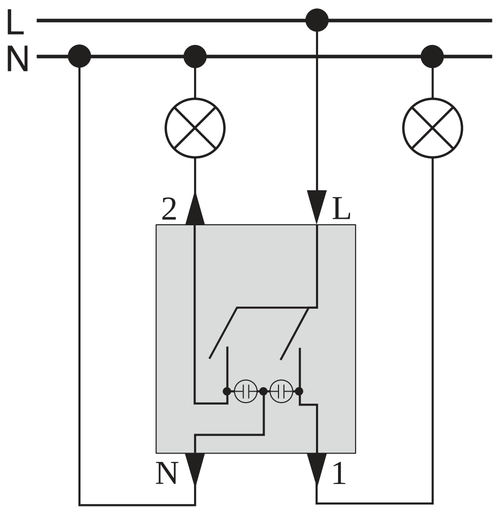
Serien-Kontrollschalter Mxx3x05-0000
