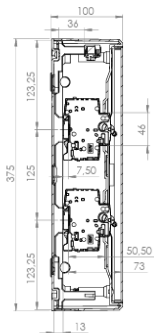
1- bis 4- reihig
