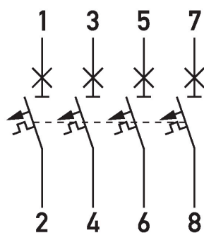
Anschlussschema DLS 6h, C-Charakteristik, vierpolig
