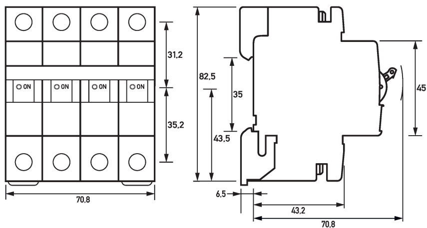
Maßzeichnung DLS 6h, C-Charakteristik, vierpolig (Gruppenansicht)
