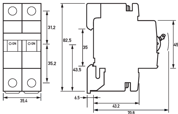
Maßzeichnung DLS 6h, C-Charakteristik, zweipolig (Gruppenansicht)
