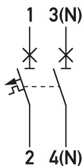
Anschlussschema DLS 6h, C-Charakteristik, einpolig+N
