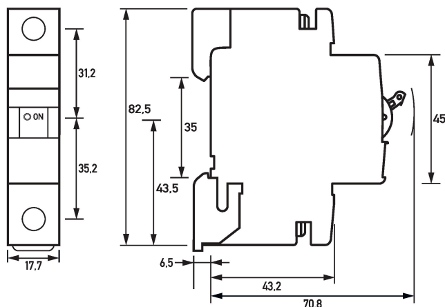
Maßzeichnung (Gruppenansicht)
