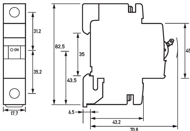
Maßzeichnung (Gruppenansicht)
