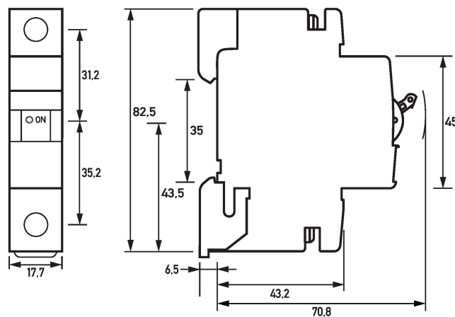
Maßzeichnung (Gruppenansicht)
