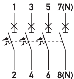
Anschlussschema DLS 6h, B-Charakteristik, dreipolig+N
