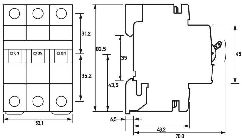
Maßzeichnung DLS 6h, B-Charakteristik, dreipolig (Gruppenansicht)
