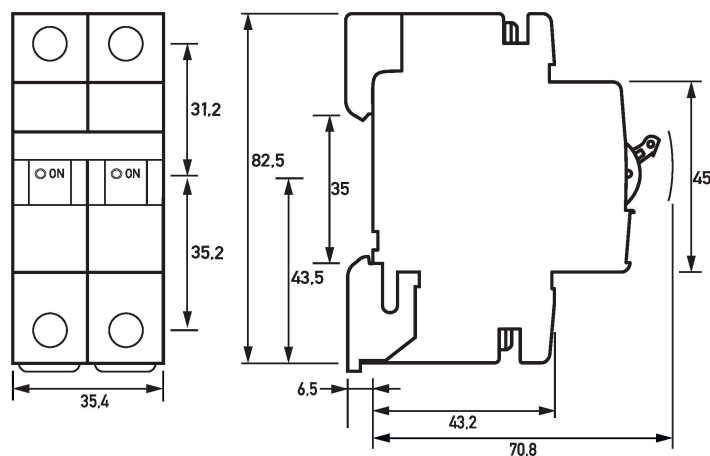
Maßzeichnung DLS 6h, B-Charakteristik, einpolig+N (Gruppenansicht)
