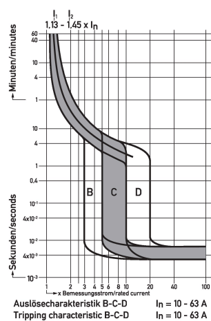
Kennlinie Char. B, C, D
