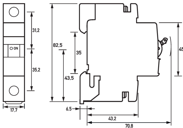
Maßzeichnung DLS 6h, B-Charakteristik, einpolig (Gruppenansicht)
