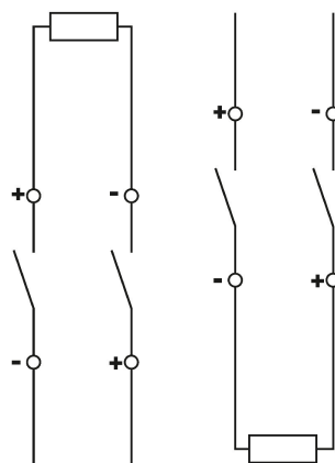
Anschlussschema DLS 6hdc, C-Charakteristik, zweipolig
