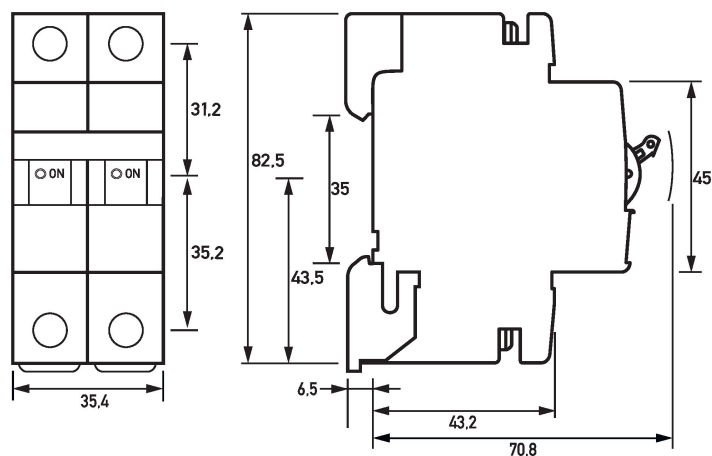
Maßzeichnung DLS 6hdc, C-Charakteristik, zweipolig (Gruppenansicht)
