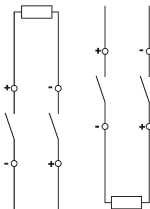
Anschlussschema DLS 6hdc, C-Charakteristik, zweipolig
