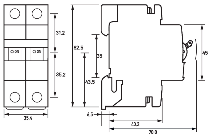
Maßzeichnung DLS 6hdc, B-Charakteristik, zweipolig (Gruppenansicht)
