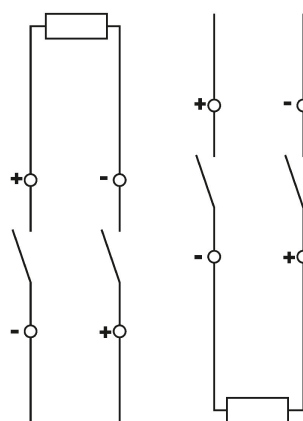
Anschlussschema DLS 6hdc, B-Charakteristik, zweipolig
