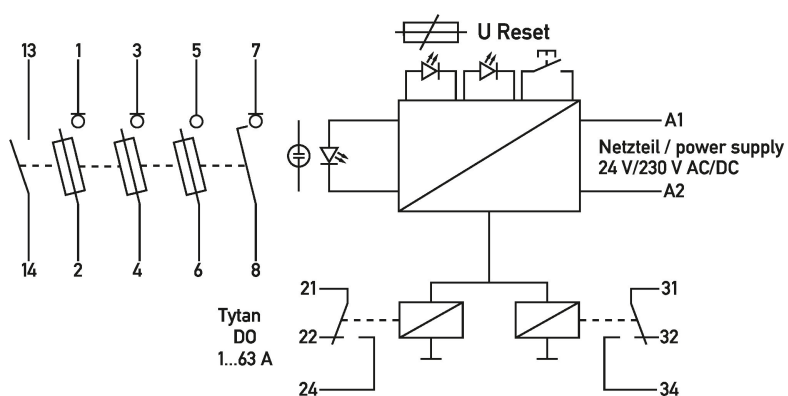
Anschlussschema Tytan mit Überwachung (Leergehäuse)
