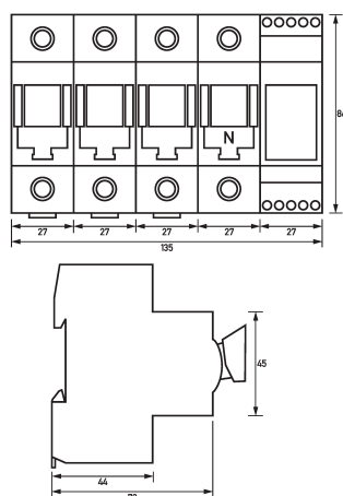
Maßzeichnung Tytan mit Überwachung (Leergehäuse) (Gruppenansicht)
