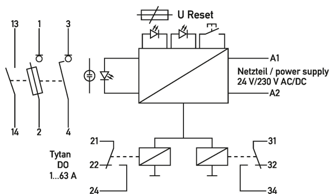
Anschlussschema Tytan mit Überwachung (Leergehäuse)
