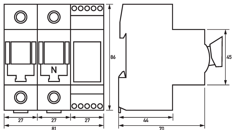
Maßzeichnung Tytan mit Überwachung (Leergehäuse) (Gruppenansicht)
