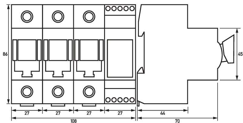
Maßzeichnung Tytan mit Überwachung (Leergehäuse) (Gruppenansicht)
