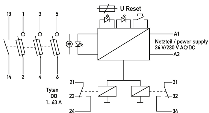
Anschlussschema Tytan mit Überwachung (Leergehäuse)
