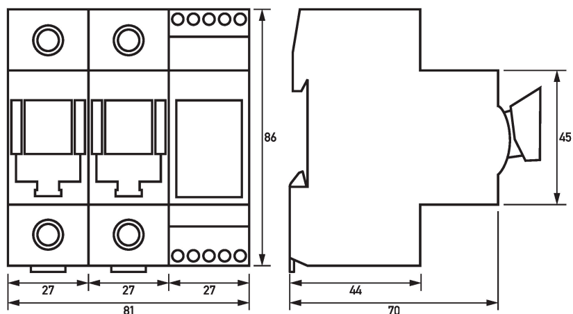
Maßzeichnung Tytan mit Überwachung (Leergehäuse) (Gruppenansicht)
