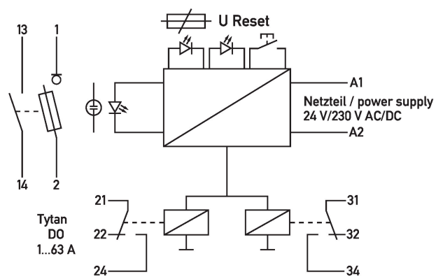
Anschlussschema Tytan mit Überwachung (Leergehäuse)
