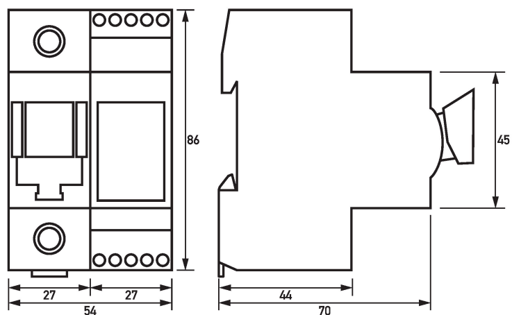
Maßzeichnung Tytan mit Überwachung (Leergehäuse) (Gruppenansicht)
