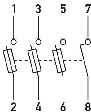
Anschlussschema Tytan verriegelbar (Leergehäuse)
