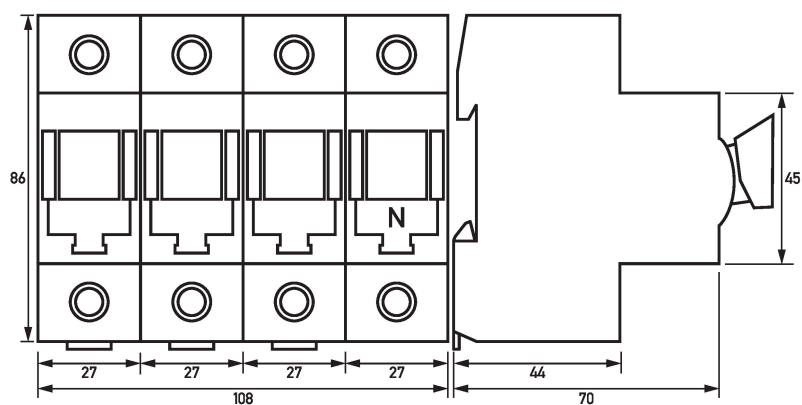
Maßzeichnung Tytan verriegelbar (Leergehäuse) (Gruppenansicht)
