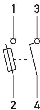
Anschlussschema Tytan (Leergehäuse)
