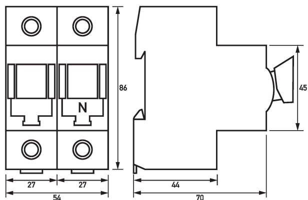
Maßzeichnung Tytan (Leergehäuse) (Gruppenansicht)
