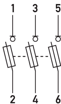
Anschlusschema Tytan (Leergehäuse)
