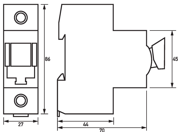
Maßzeichnung Tytan (Leergehäuse) (Gruppenansicht)
