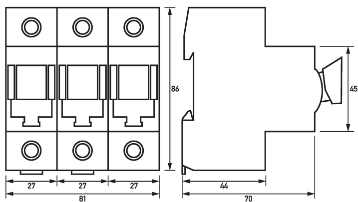
Maßzeichnung Tytan (Gruppenansicht)
