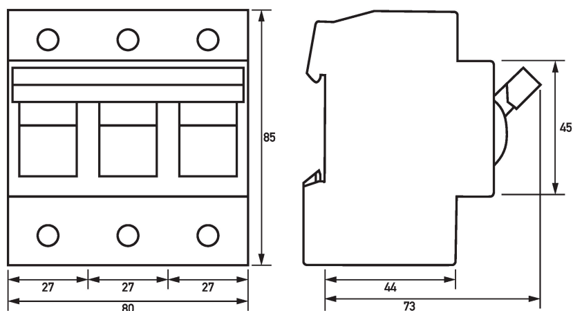
Maßzeichnung Coron 2 (Gruppenansicht)
