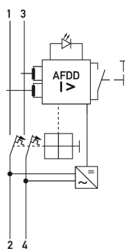
Anschlussschema DAFDD 1 Typ A, 2-polig
