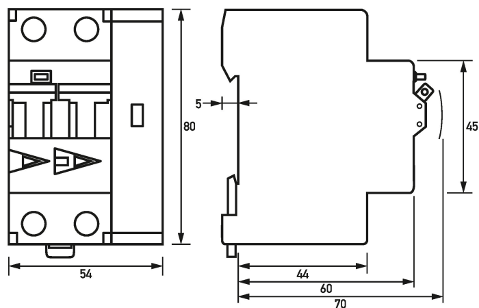
Maßzeichnung DAFDD 1 Typ A, 2-polig (Gruppenansicht)
