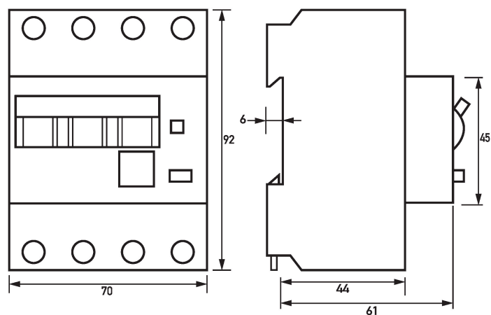
Maßzeichnung DRCBO 4 Typ A, 3+N-polig (Gruppenansicht)
