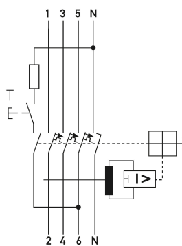
Anschlussschema DRCBO 4 Typ A, 3+N-polig
