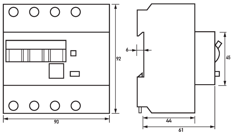
Maßzeichnung DRCBO 4 Typ A, 3+N-polig (Gruppenansicht)
