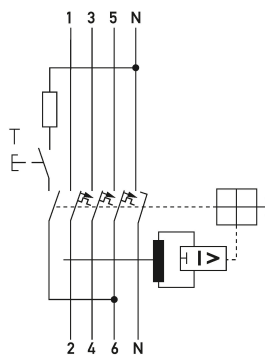
Anschlusschema DRCBO 4 Typ A, 3+N-polig
