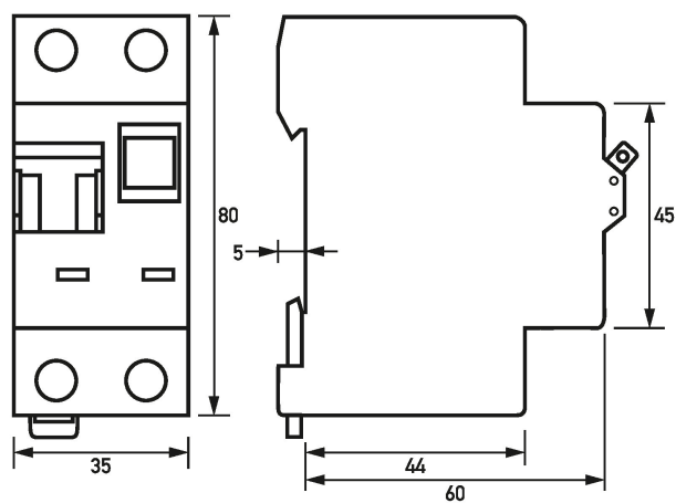
Maßzeichnung (Gruppenansicht)
