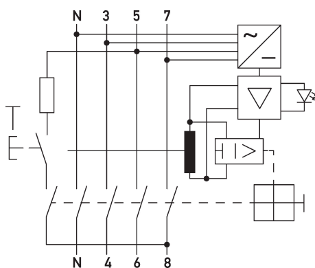
Anschlussschema DFS 4 B SK, 4-polig
