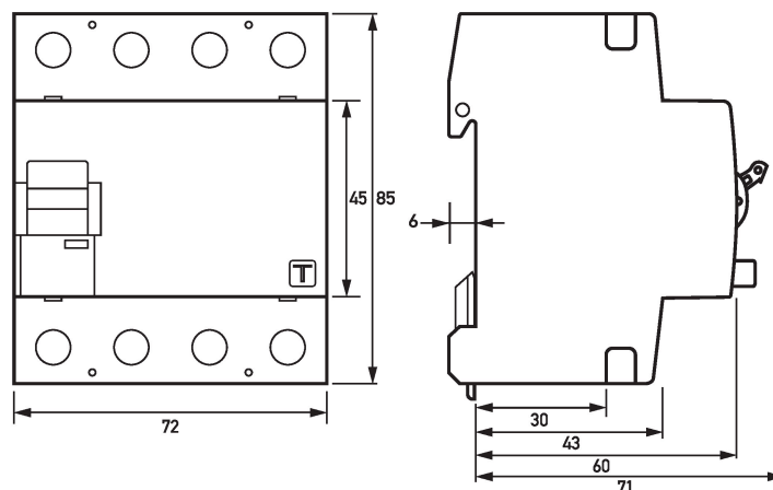
Maßzeichnung DFS 4 B SK, 4-polig (Gruppenansicht)
