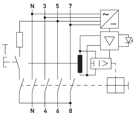
Anschlusschema DFS 4 B NK, 4-polig
