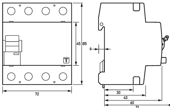
Maßzeichnung DFS 4 B NK, 4-polig (Gruppenansicht)
