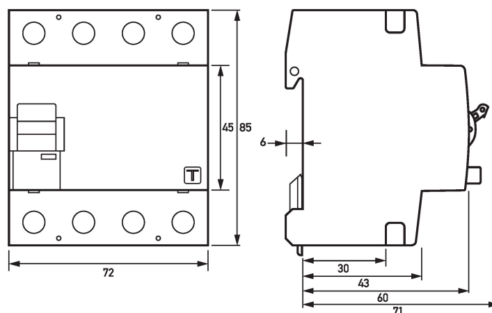
Maßzeichnung DFS 4 F, 4-polig (Gruppenansicht)
