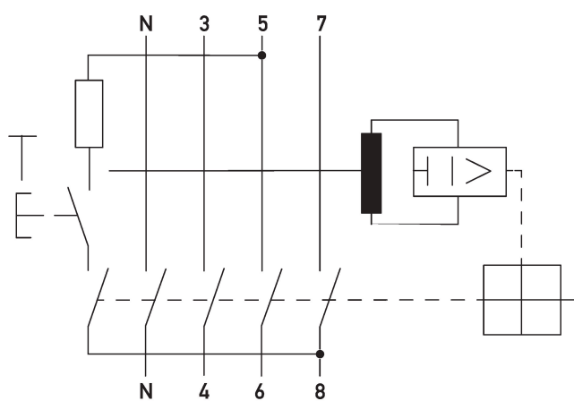
Anschlussschema DFS 4 F, 4-polig
