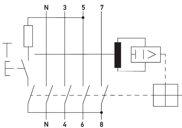
Anschlussschema DFS 4 A, 4-polig
