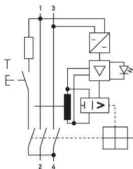
Anschlussschema DFS 2 B SK, 2-polig
