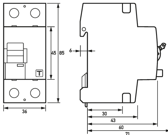
Maßzeichnung DFS 2 B SK, 2-polig (Gruppenansicht)
