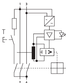
Anschlusschema DFS 2 B SK, 2-polig
