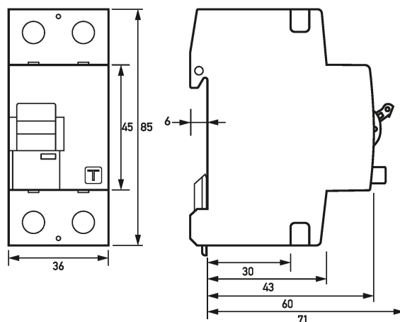
Maßzeichnung DFS 2 B NK, 2-polig (Gruppenansicht)
