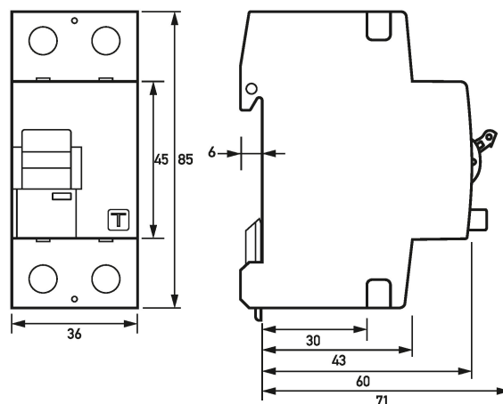
Maßzeichnung DFS 2 F, 2-polig (Gruppenansicht)
